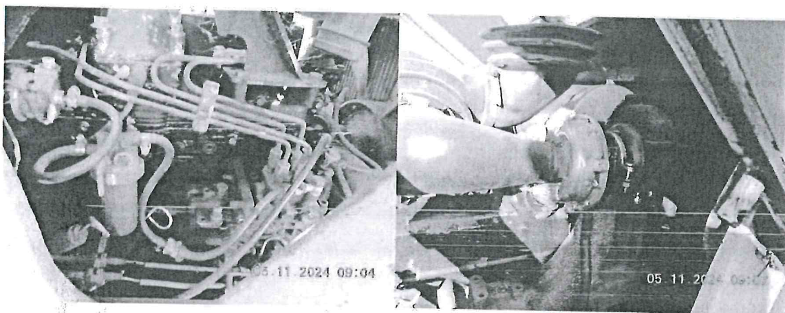
Foto. 3 Imagine cu grupul propulsor al MAL – ului evaluat.
