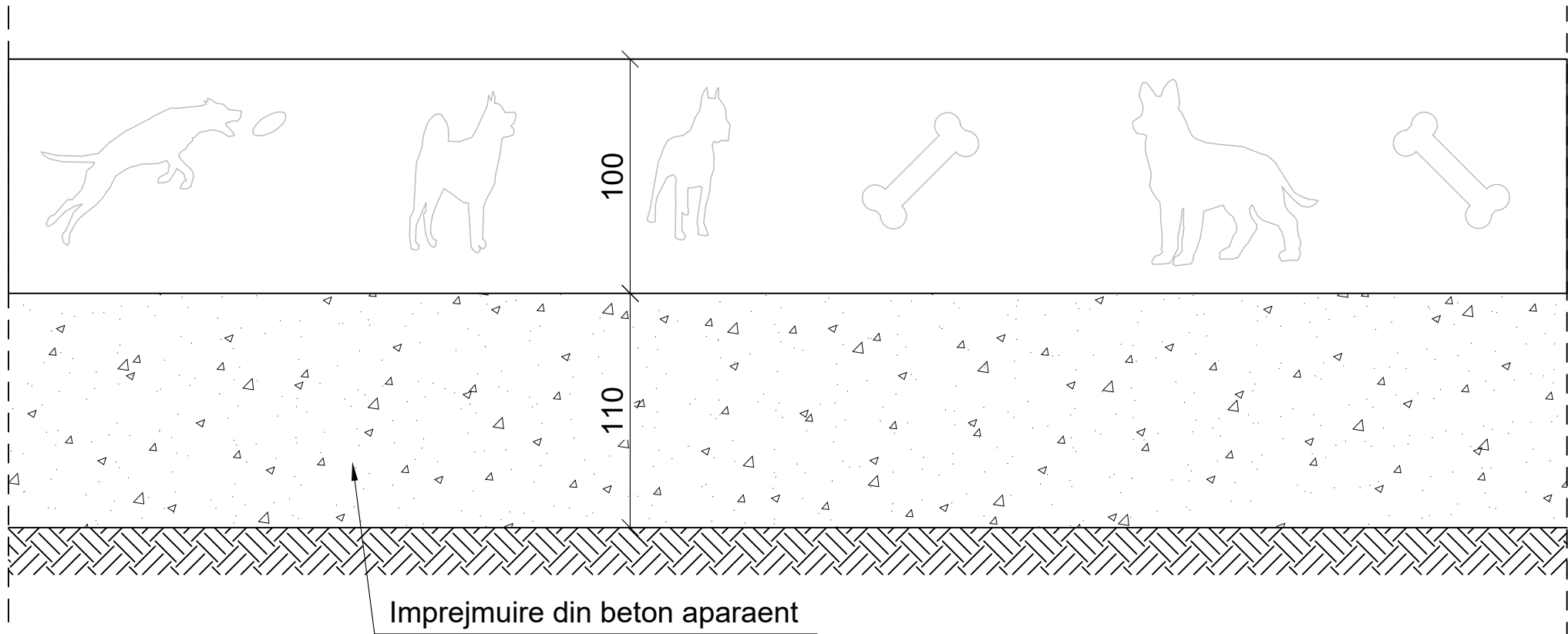
Sectiune transversala
