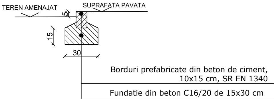
Detalii realizare borduri
