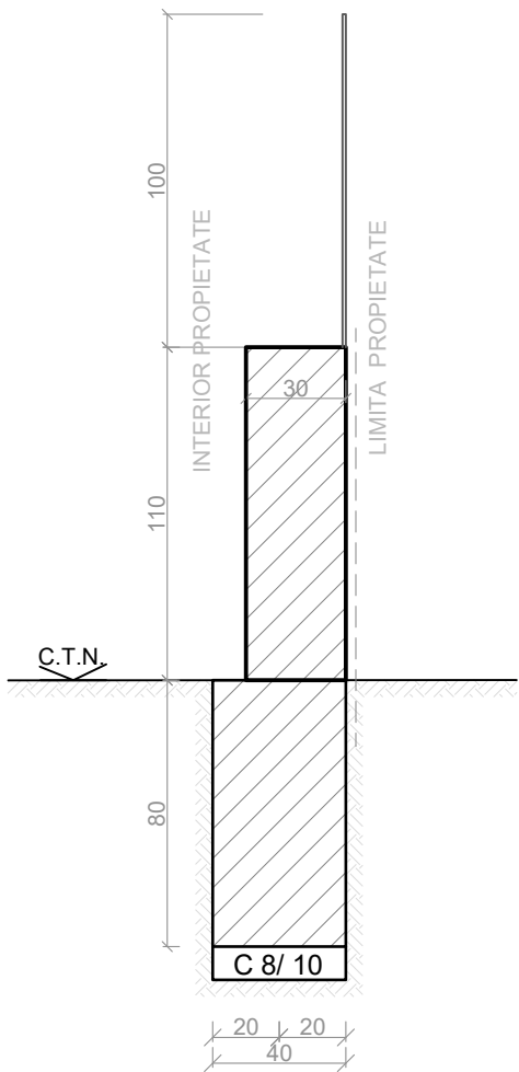
Sectiune transversala
