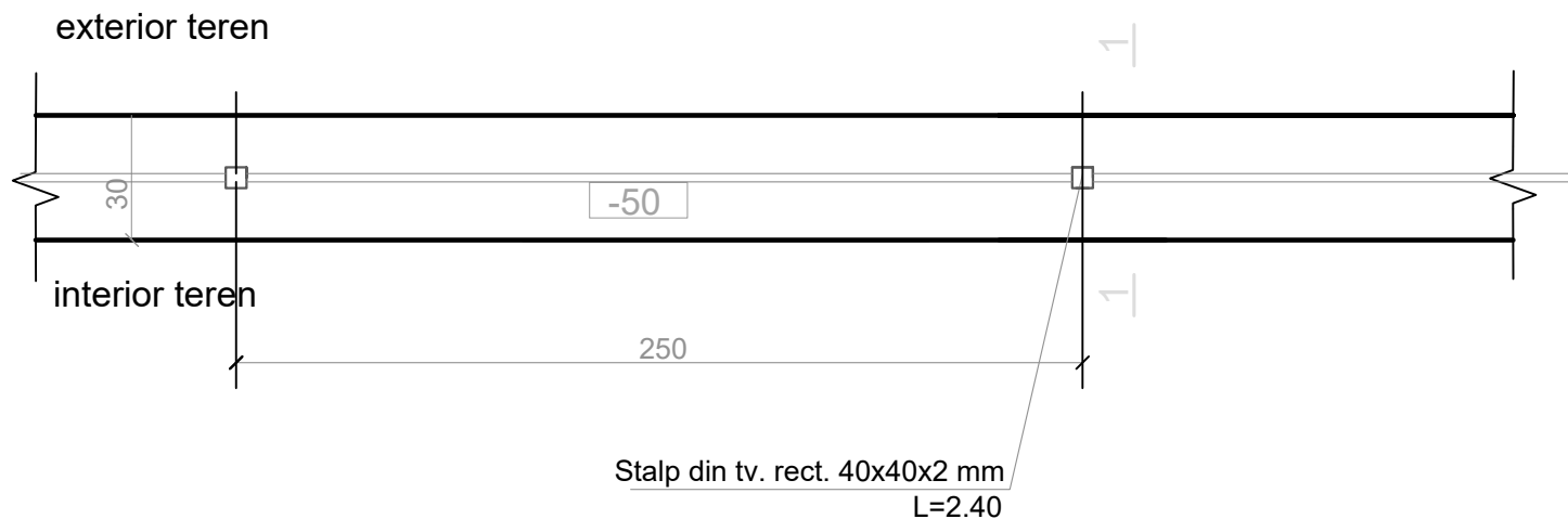
PLAN FUNDATII scara 1:20
