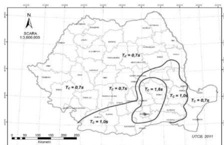
Zonarea teritoriului României în termeni de perioadă de control (cicl), T_c , a spectrului de răspuns
