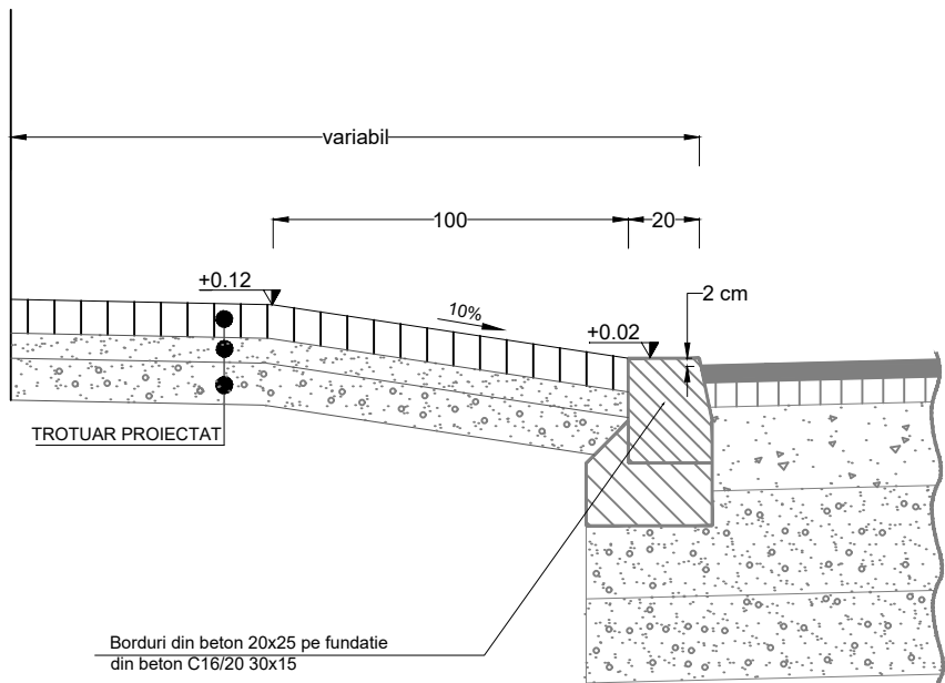
SECTIUNE C-C Sc: 1:20
