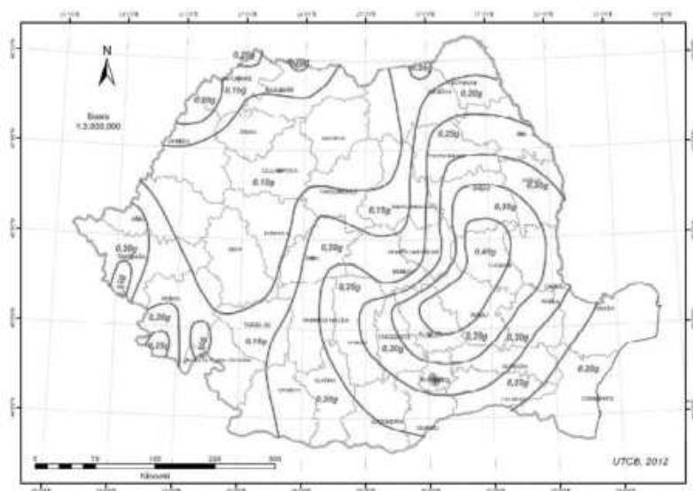
Zonarea teritoriului României în termeni de valuri de vârf ale accelerației terenului pentru proiectare ag pentru cutremure având intervalul mediu de recurență IMR = 225 ani și 20% posibilitate de depășire în 50 de ani.
