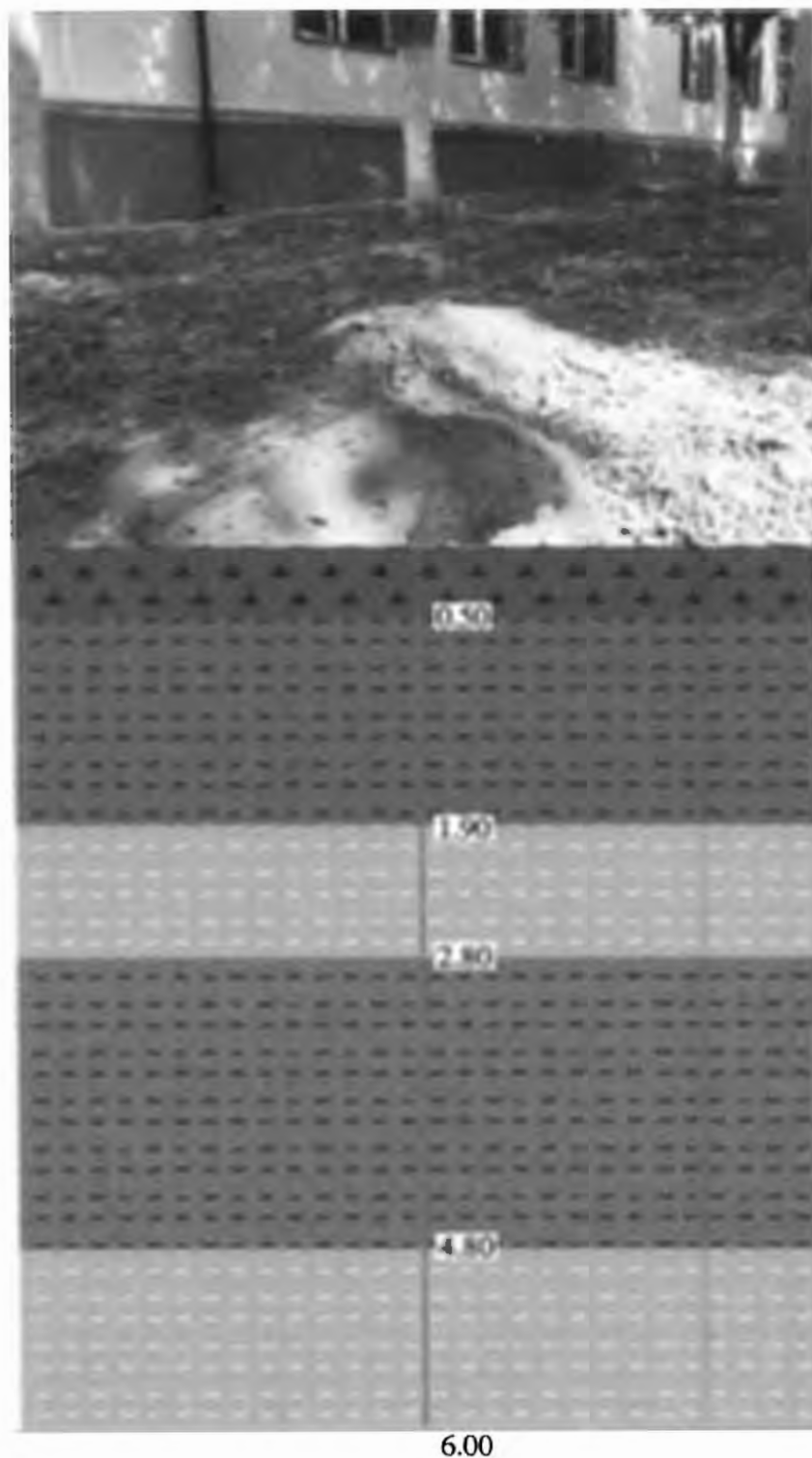
Argila prafoasa - praf argilos cafeniu deschis, cu calcar fin diseminat, plastic vartos
