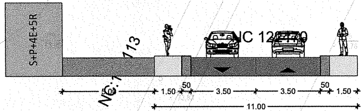
SECTIUNE A-A' - Str. Echinocitului scara 1:200
